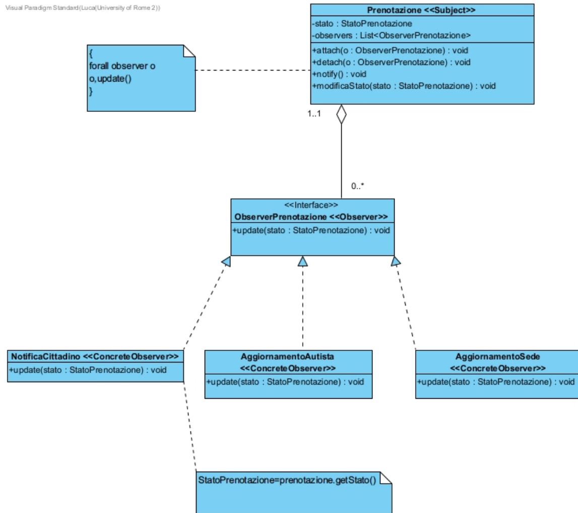
Figura 46: Struttura UML del Design Pattern Observer applicato a MyAma
